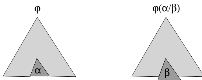
Abbildung 1.1: Sind \alpha und \beta äquivalent, so auch \varphi und \varphi(\alpha/\beta) .
